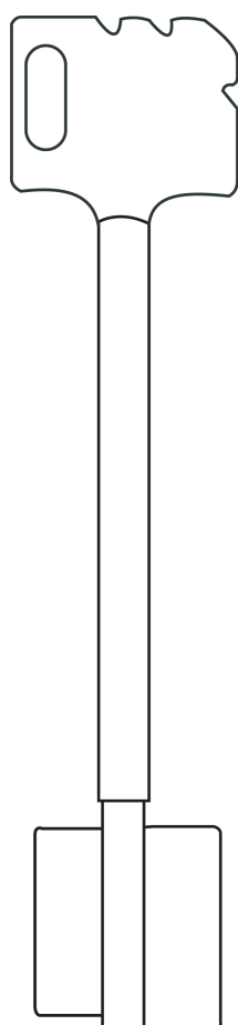
MAU5A 118 mm ø INT 3.5 ø EXT 6.8
